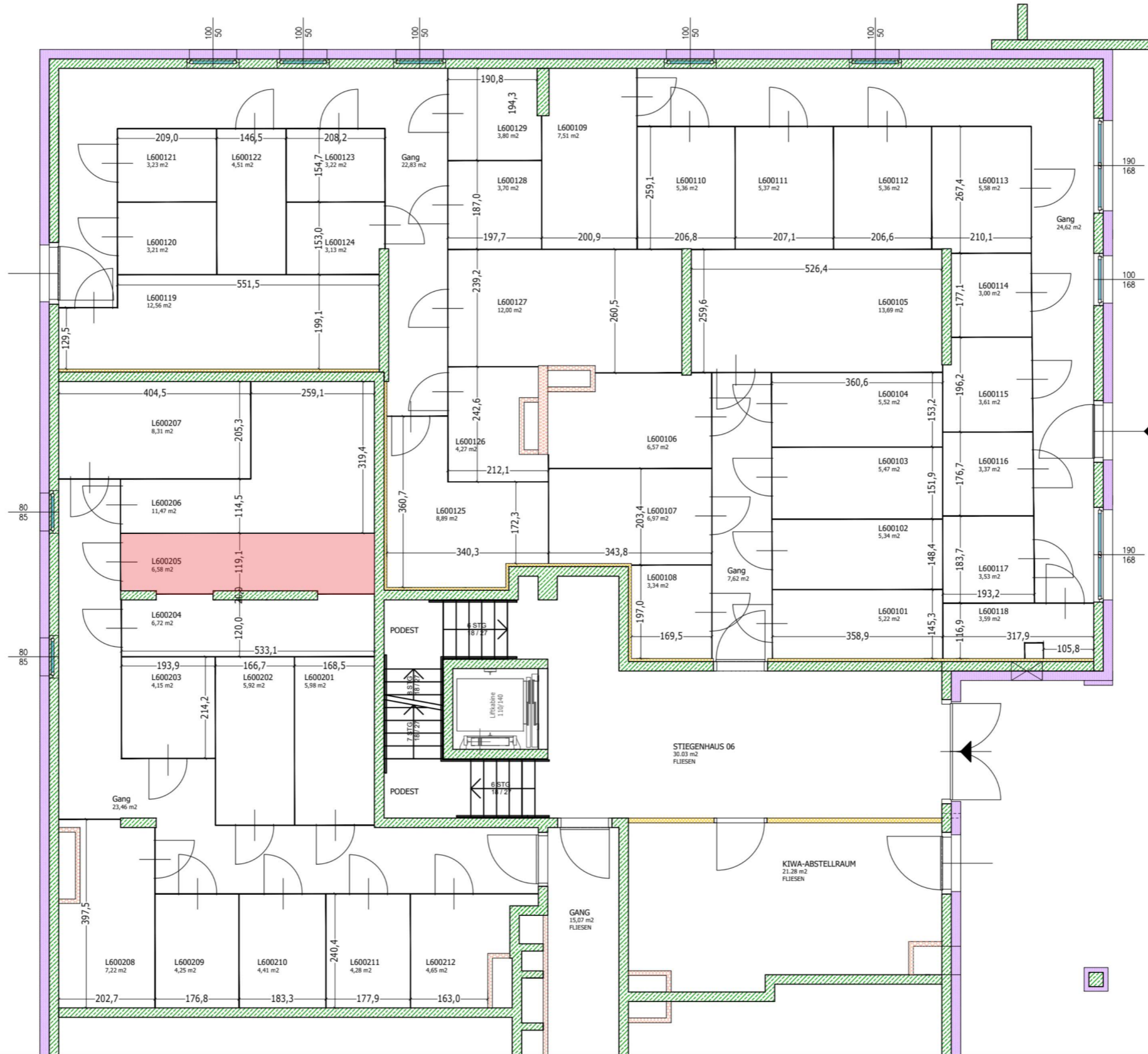
WOHNPAK DERPUNKT - STIEGE 06 GRUNDRISS ERDGESCHOSS M1:100 LAGERAUFTEILUNG 02.06.2023
