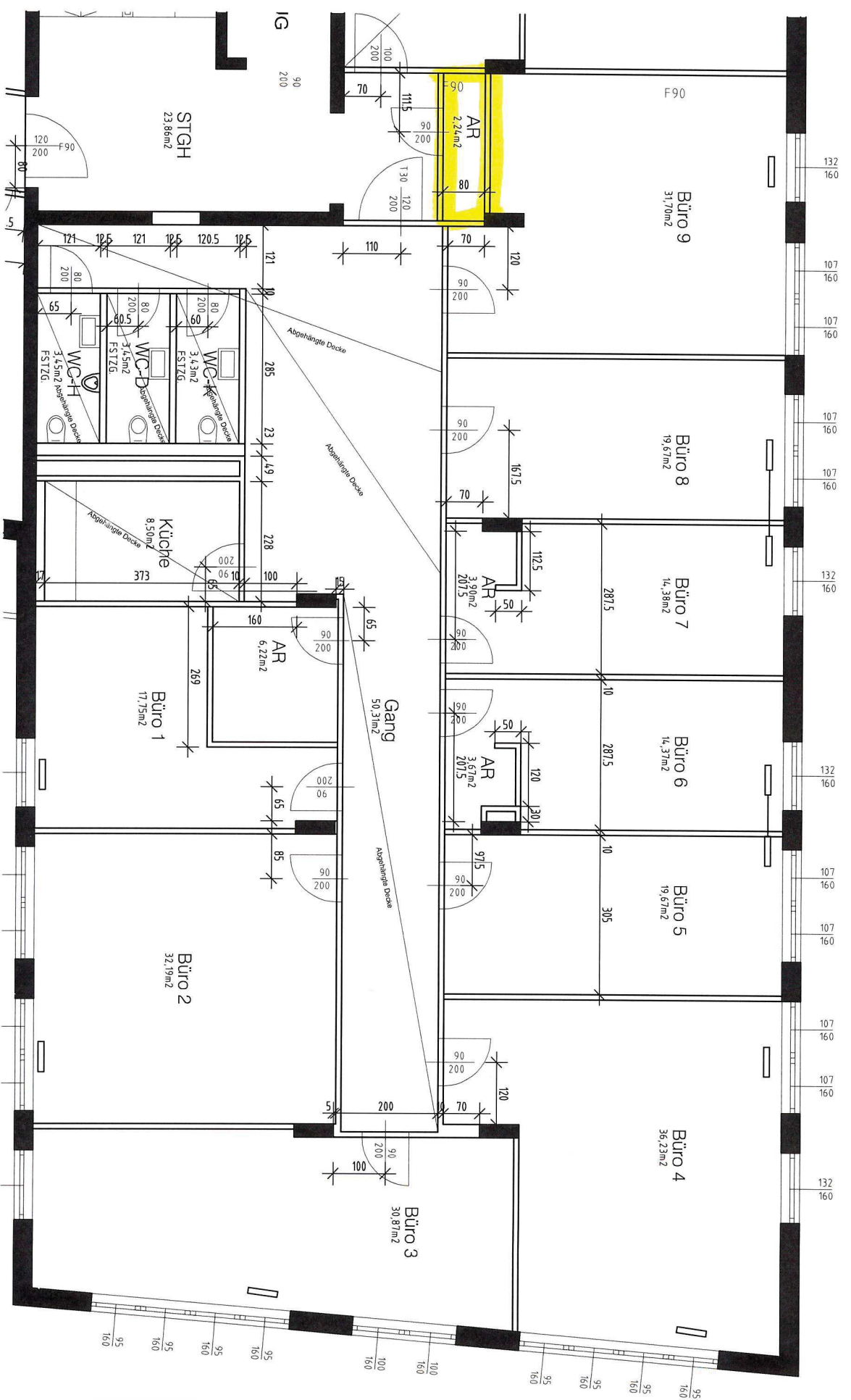
GRUNDRISS 3.OG BAUTEIL IV AUSFÜHRUNGSPLAN 1:100
