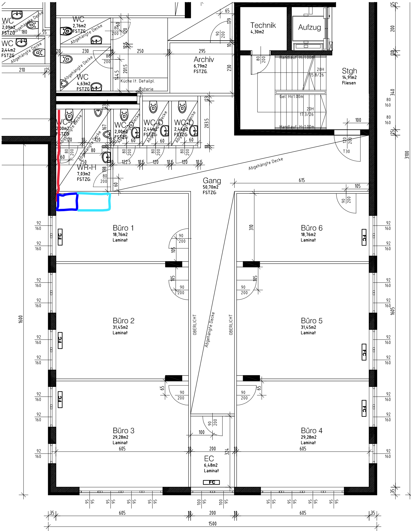
GRUNDRISS 2.OG STIEGE J BAUTEIL II - AUSFÜHRUNGSPLAN 1:1
